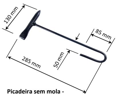
Picadeira sem mola - Cód. 2061
