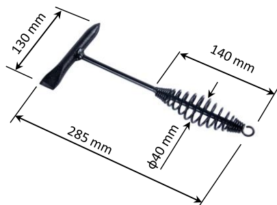
Picadeira com mola - Cód. 2060
